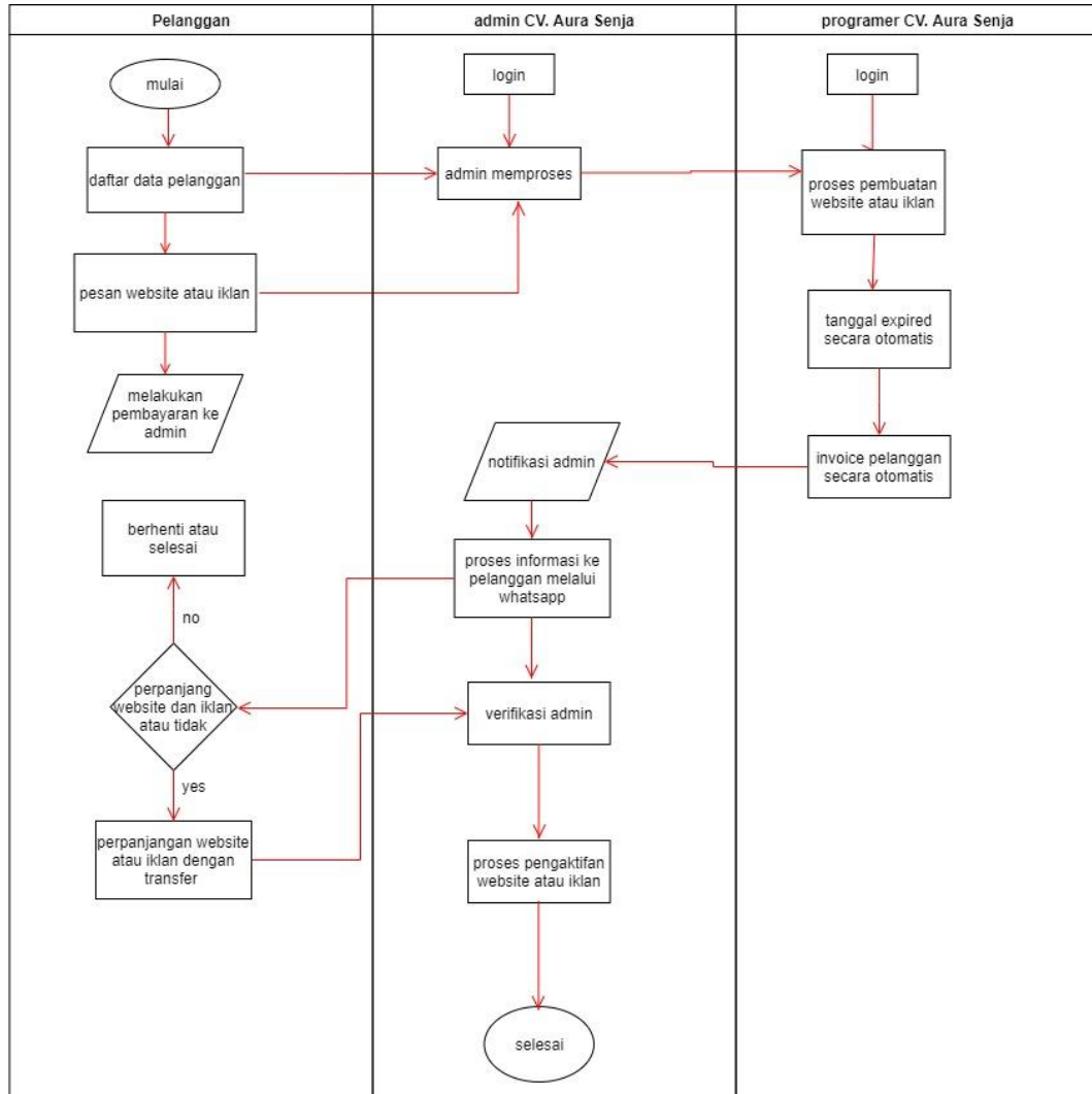
Gambar 3.1 Bisnis Proses
