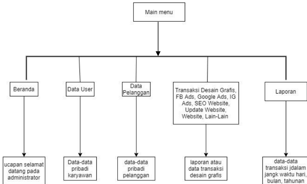
Gambar 4.1. Struktur Menu
