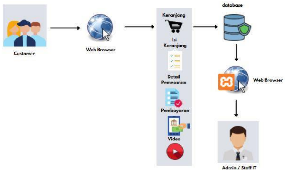
Gambar 3.1 Desain Sistem / Arsitektur Sistem
