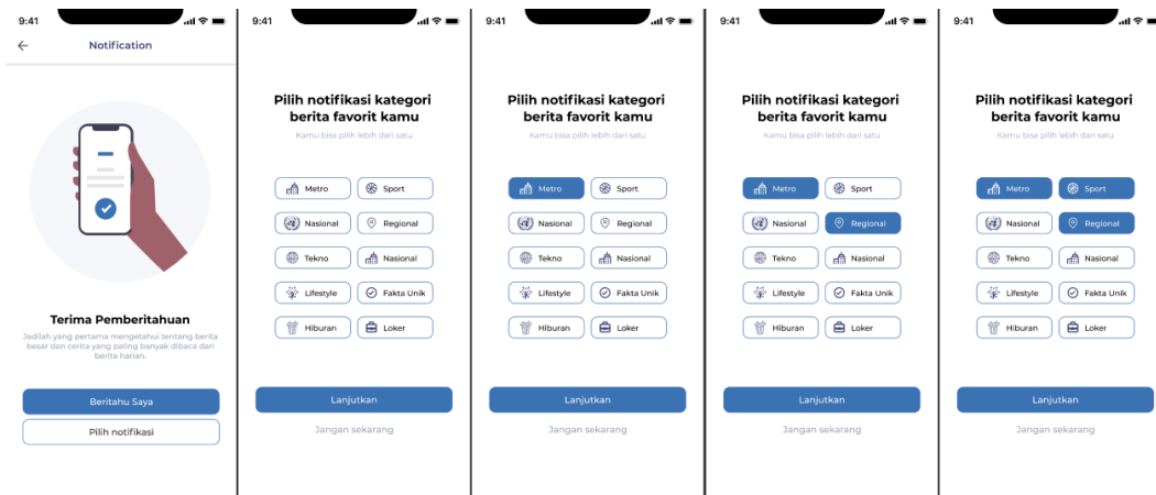
Gambar 5. 5 Purwarupa halaman pilih Kategori Notifikasi
