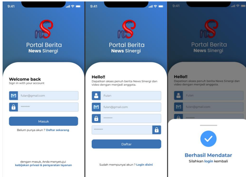
Gambar 5. 2 Purwarupa halaman Register dan Login
